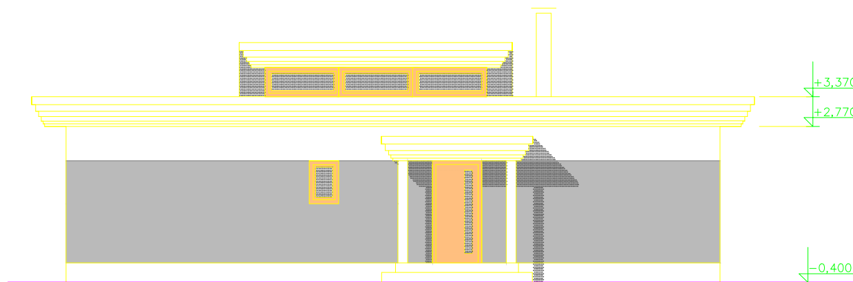
pohled severní
